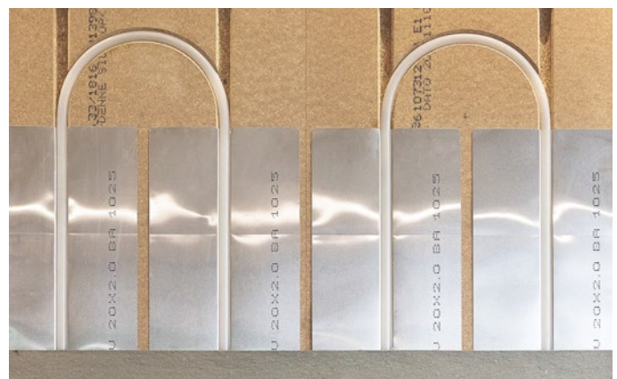
Figur 3 Värmefördelningsplattor speciellt utvecklade för 38 mm Klimagolv.
